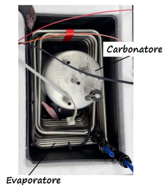
Banco ghiaccio aperto, vista dall'alto
