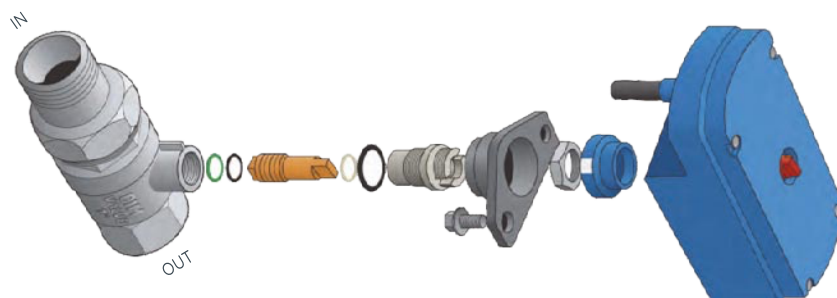
Esploso valvola a sfera con attuatore elettrico
