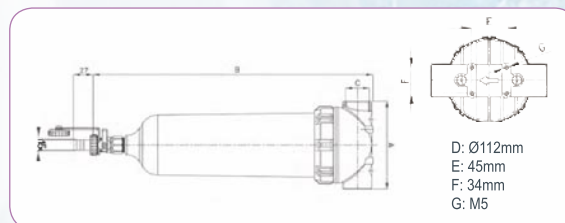
F03 vaso SAN trasparente-trogamid-opaco bianco
