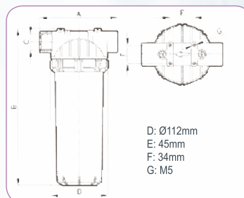
F03 vaso SAN trasparente-trogamid-opaco bianco
